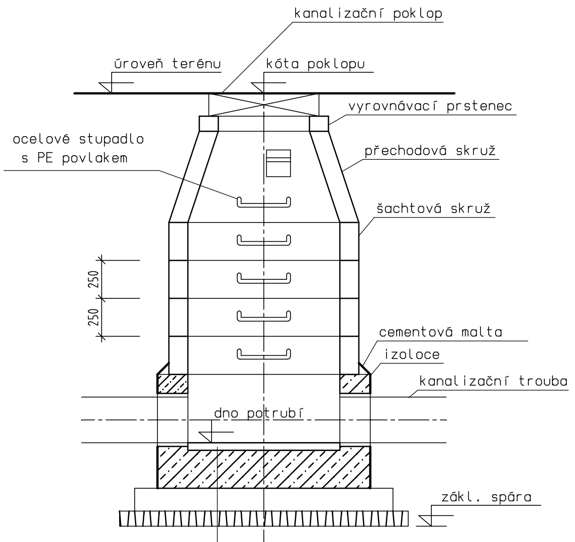
Podélný řez
